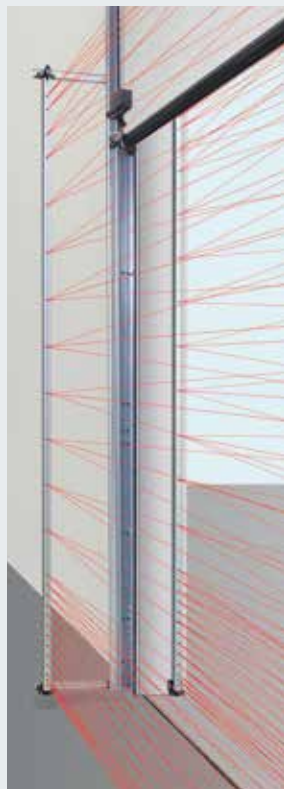
Lichtgitter HLG für Schlupftür Tore
