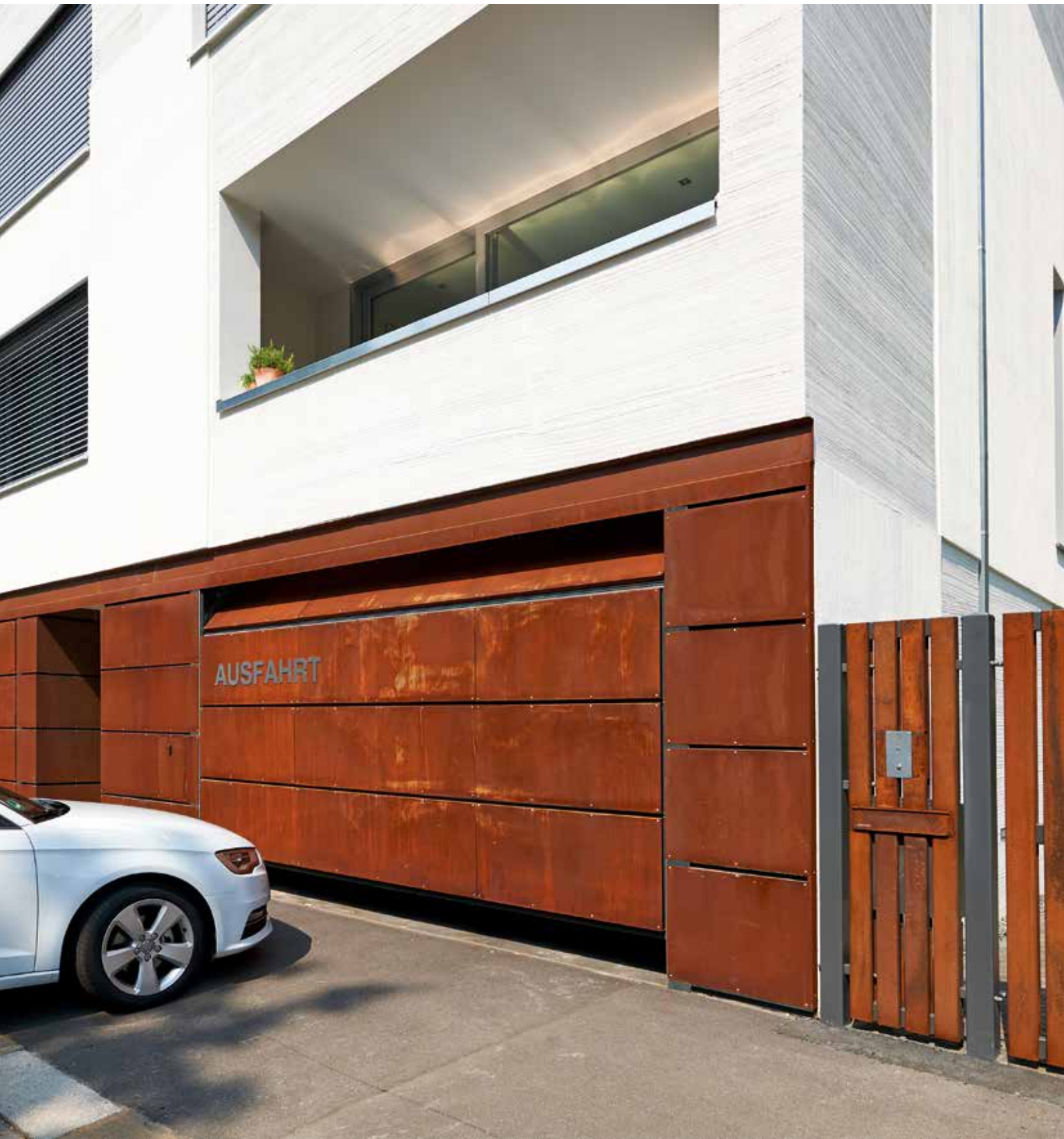
Bauseitige Beplankung mit Schichtpressplatten
