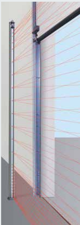
Lichtgitter HLG-V Montage mit Standsäulen-Set STL
